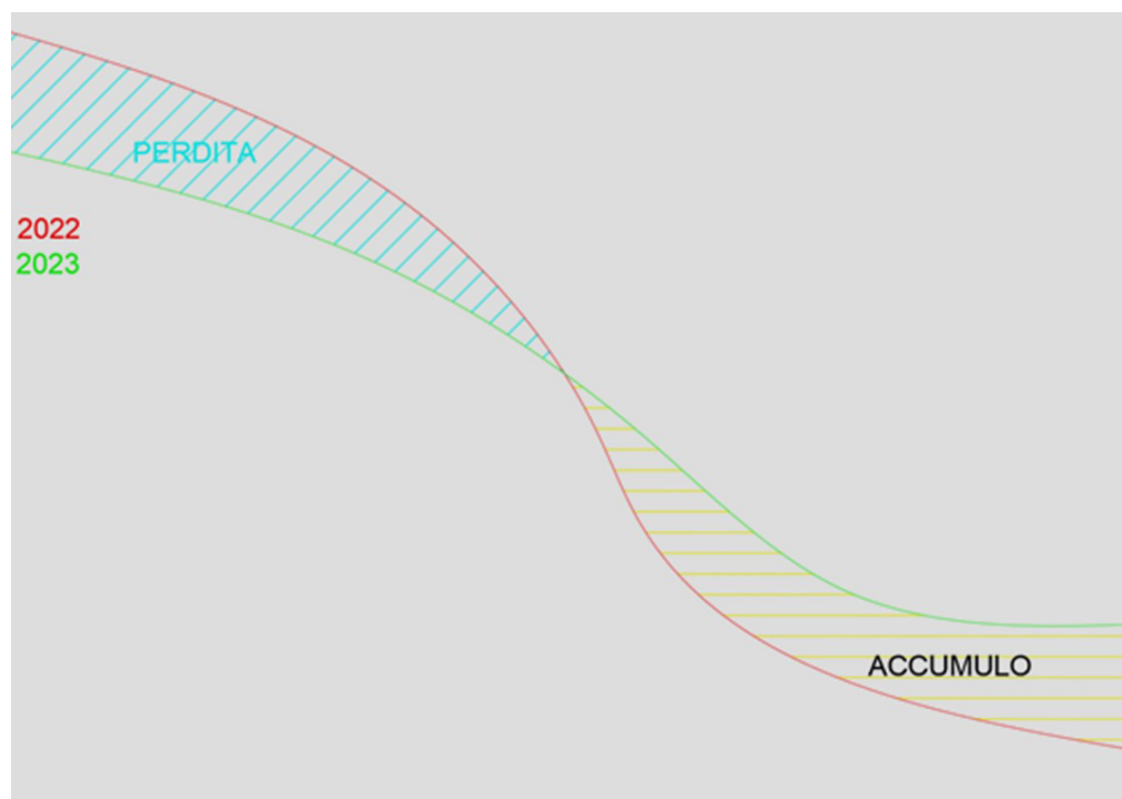
Fig. 7 - Sezione tipo, schematica, della nuova metodologia proposta a «contenitore geomorfologico invariato», in cui sono riportate le tracce delle due superfici relative a due annate dell'anno idrologico di bilancio. Il calcolo dei volumi è effettuato attraverso il confronto tra le intersezioni delle due superfici. Schematic type section of the proposed new methodology with an "unchanged geomorphological container," showing the traces of the two surfaces corresponding to two years of the hydrological balance year, with volume calculation performed by comparing the intersections of the two surfaces.
