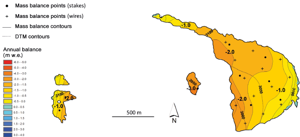
FIG. MB9 - Distribuzione spaziale del bilancio annuale sul ghiacciaio del Careser nel 2019. Annual balance distribution on the Careser Glacier in 2019.
