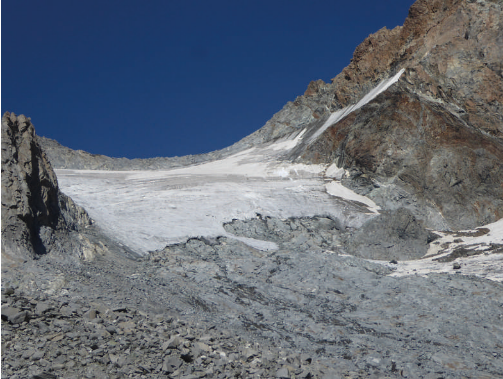
408 - Ghiacciaio di Predarossa; stazione fotografica SF245 (foto M. URSO, 2019.09.21). La neve residua dell'anno è molto ridotta e si accumula solamente alla base delle pareti rocciose. Annual residual snow is very reduced and accumulated at the toe of rocky walls.
