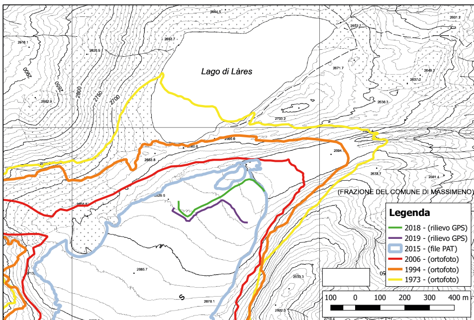
634 - Ghiacciaio di Lâres. Variazione della posizione planimetrica del margine frontale a partire dal 1973 (elaborazione M. VALENTINI). Variation of the planimetric position of the frontal margin from 1973.
