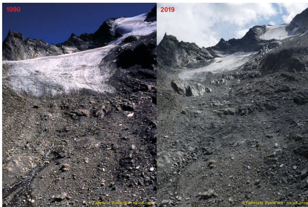
159 - Ghiacciaio di L'Espine (foto F. POLLICINI, 2019.08.30 e 1990.08.19). Dal 1990 ad oggi il ghiacciaio si è considerevolmente ridotto, frammentandosi in due corpi distinti, in corrispondenza di un gradino roccioso. From 1990 to today, the glacier has considerably shrunk, fragmenting into two distinct bodies, in correspondence with a rock step.
