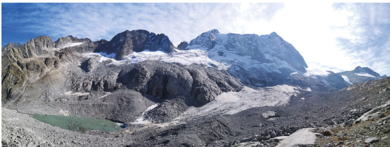
678 - Ghiacciaio della Presanella; stazione fotografica SF19 (foto C. FERRARI, 2019.09.29). La fronte del ghiacciaio si affaccia sul lago proglaciale che si è formato a metà degli anni '90. Il settore frontale del ghiacciaio rimane collegato al corpo superiore solo in due punti in corrispondenza del salto roccioso. Evidente la grande morena a nucleo di ghiaccio in sinistra idrografica. The front of the glacier overlooks the proglacial lake that formed in the mid-1990s. The frontal sector of the glacier remains connected to the upper body only in two points along the rocky step. A large ice-core moraine rise on the hydrographic left.
