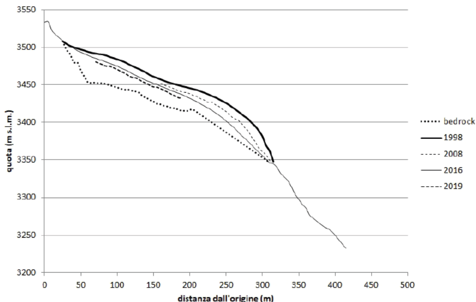
Ghiacciaio della Croce Rossa: sezione SW-NE
