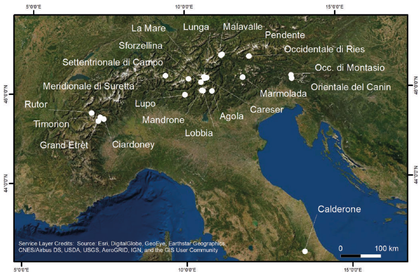
FIG. MB1 - Collocazione geografica dei ghiacciai italiani per i quali si riportano i valori di bilancio di massa nell'anno 2019. Geographic setting of the Italian mass balance glaciers with reported data for 2019.
