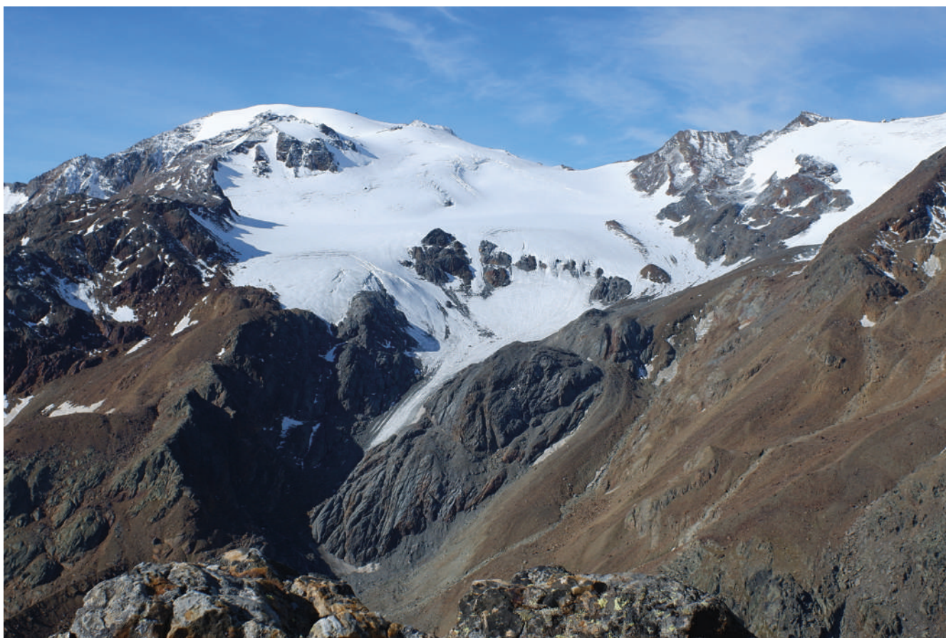
FIG. MB5 - Il ghiacciaio de La Mare ripreso il 27 settembre 2019 da cima Nera (foto L. CARTURAN). Il ghiacciaio è ricoperto da un sottile strato di neve recente. The La Mare Glacier photographed from Cima Nera on 27 September 2019. A thin layer of fresh snow covers the glacier.
