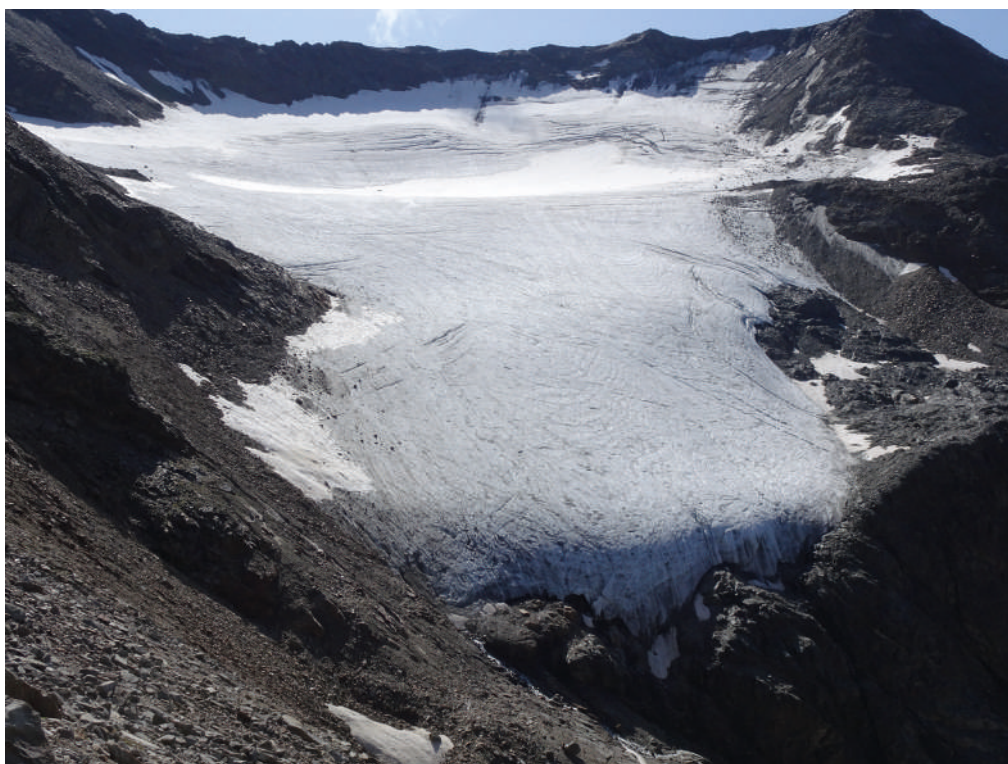
754 - Ghiacciaio di Rosim - Rosimferner (foto G. BARISON, 2019.08.22). Si osservano diversi crolli di detrito, specie sul fianco sinistro del bacino superiore. L'ablazione particolarmente pronunciata evidenzia le foliazioni del ghiacciaio. Sono ancora presenti numerose placche di neve vecchia primaverile a diverse quote. Several debris collapses occurred, especially on the left flank of the upper basin. The particularly marked ablation highlights the foliation of the glacier. There are still numerous patches of old spring snow at different altitudes.
